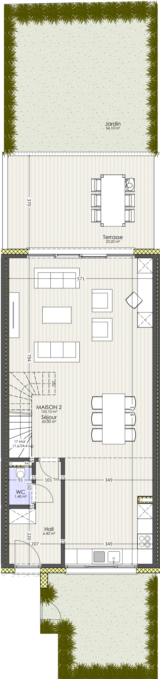
REZ-DE-CHAUSSEE
