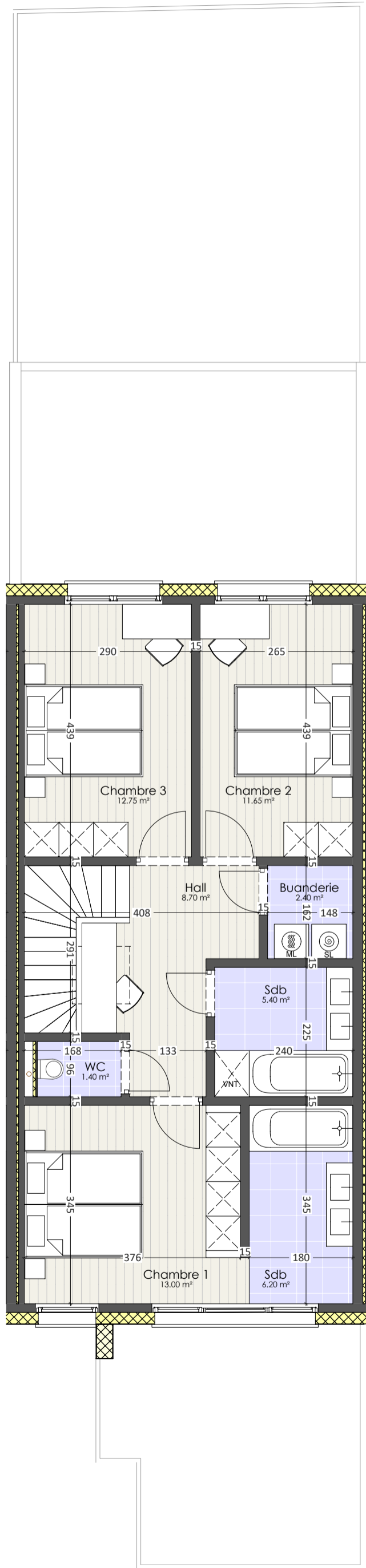
PREMIER ETAGE
