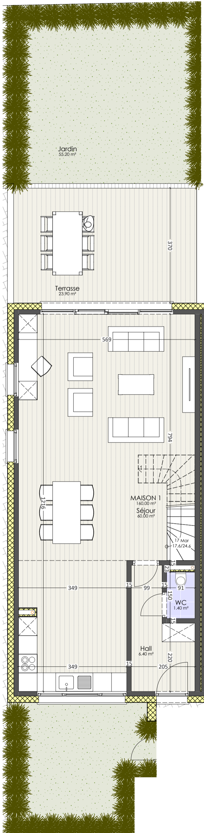
REZ-DE-CHAUSSEE
